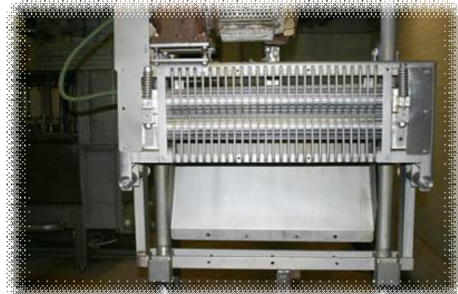
vytahovač křídelních brk
